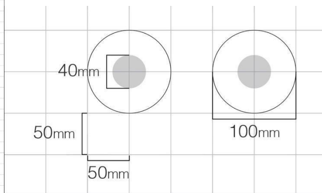
Рис. 3. Размеры элементов соревновательного полигона
